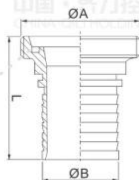
DIN软管接头 DIN hose adapter
