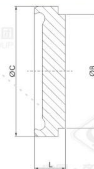
DIN/ISO/IMPERIAL - 14 LINER BLANK CAP
