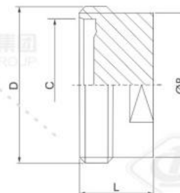
DIN/ISO/IMPERIAL - 14 LINER BLANK CAP
